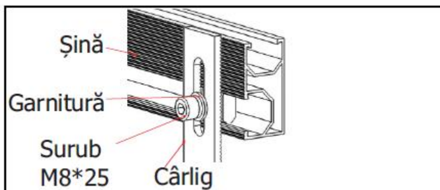
Fig. 2 - Clema HOOK - instalare
