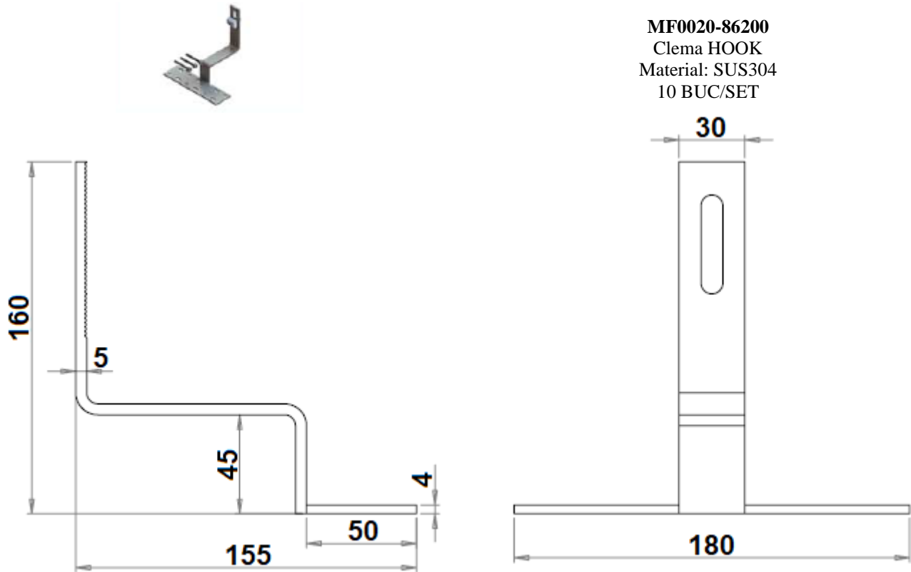
Fig. 1 - Clema HOOK - dimensiuni
